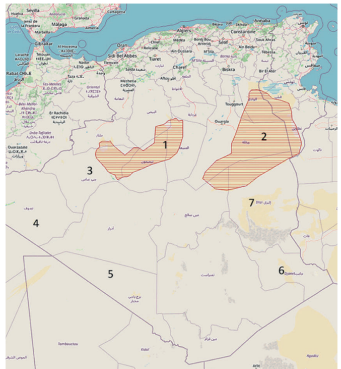
Figure 5 : Aire de répartition confirmée de G. leptoceros en Algérie (hachuré rouge) and les ergs principaux. 1. Grand erg occidental ; 2. Grand erg oriental ; 3. Erg Er Raoui; 4. Erg Iguidi; 5. Erg Chech; 6. Erg Admer; 7. Erg Issaouane.
