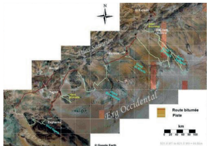
Figure 6 : Itinéraires de suivi, Grand erg occidental, 2009 (De Smet et al. 2009).
