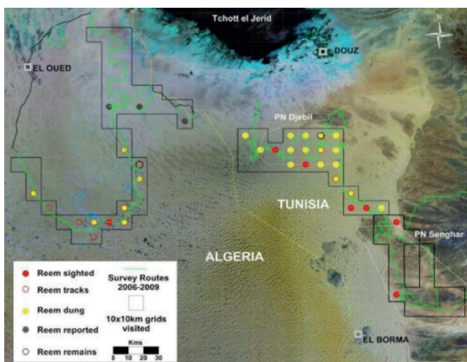
Figure 9. Localisation des observations et traces de G. leptoceros dans le Grand Erg Oriental 2006-2009 : région d'El Oued (Algérie) : P.N. de Jbil et de Senghar-Jabbes (Tunisie) (Wacher et al. 2011).
