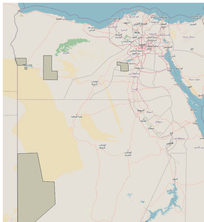
Figure 11 : Égypte et les principales localités mentionnées. 1. A.P. de Siwa ; 2. A.P. de la dépression d'El Qattara ; 3. A.P. de Wadi El Rayan ; 4. P.N. de Gilf El Kebir. 5. Oasis de Farfara (non-protégée). Polygones des A.P. selon UNEP-WCMC et IUCN (2020).
