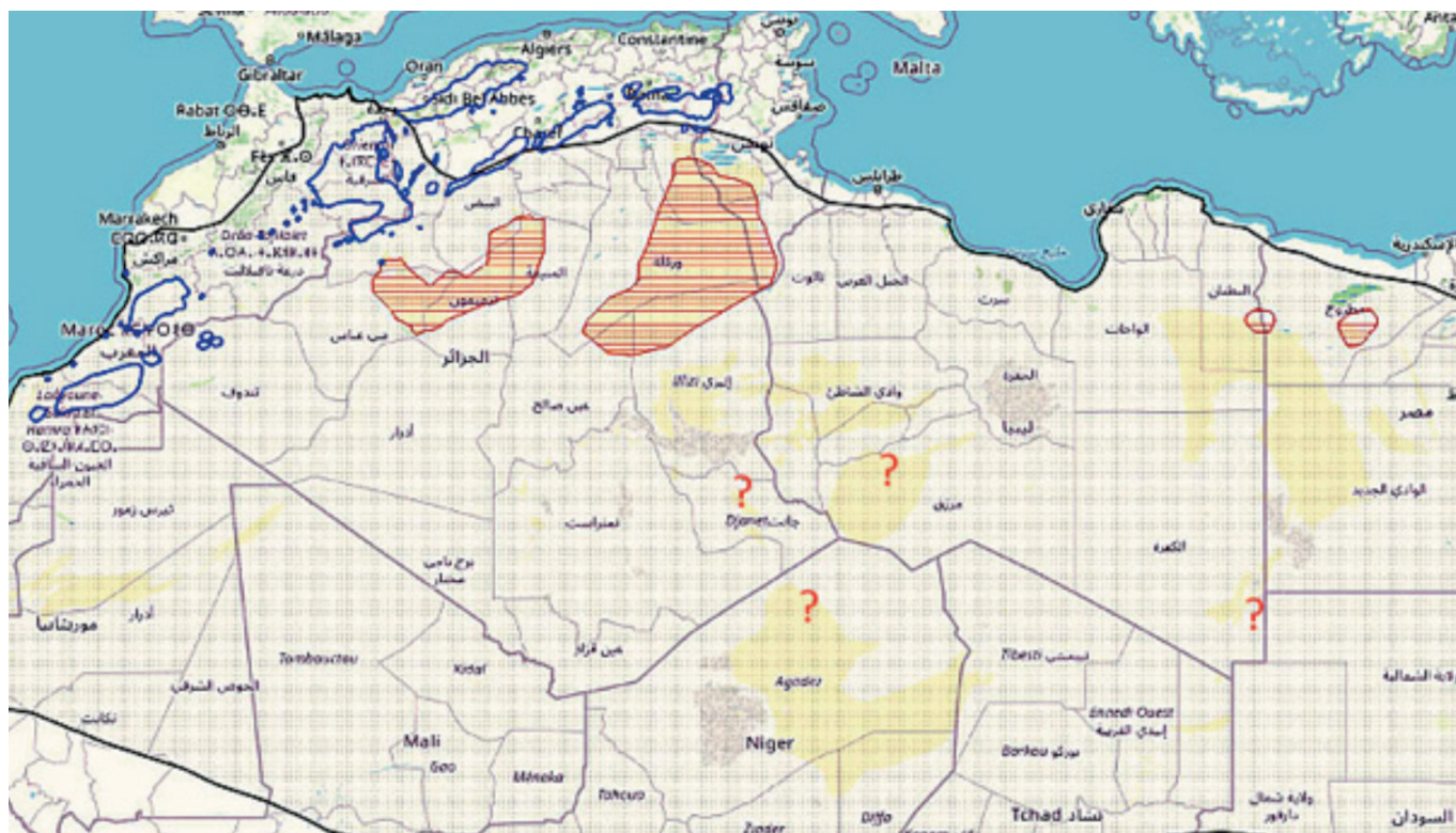
Figure 1 : Répartition récente de Gazella leptoceros (en rouge); G. cuvieri (en bleu) et G. dorcas (ligne noir) en Afrique de Nord. Les cartes de G. cuvieri et G. dorcas sont basées sur la Liste Rouge de l'IUCN ( www.iucnredlist.org )
