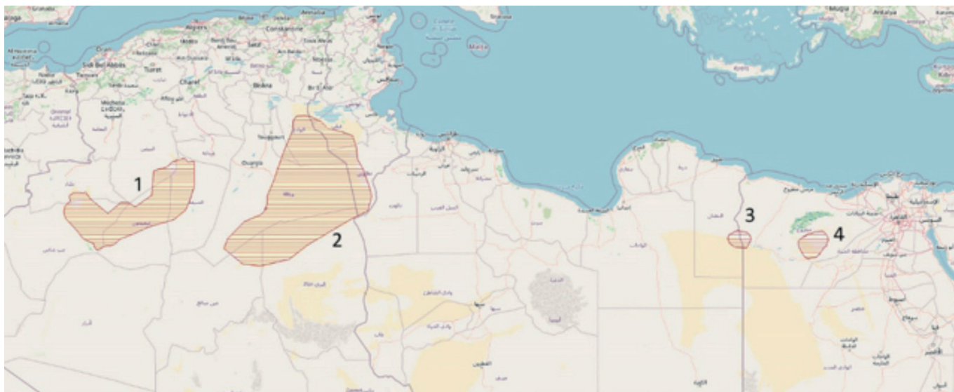
Figure 4 : Afrique du Nord : les principales zones dunaires (en jaune) ; sites où la présence de G. leptoceros a été confirmée 1990-2020 (hachuré rouge). 1. Le Grand erg occidental ; 2. Grand erg oriental ; 3. Siwa-Jaghboub ; 4. Dépression de Qattara.
